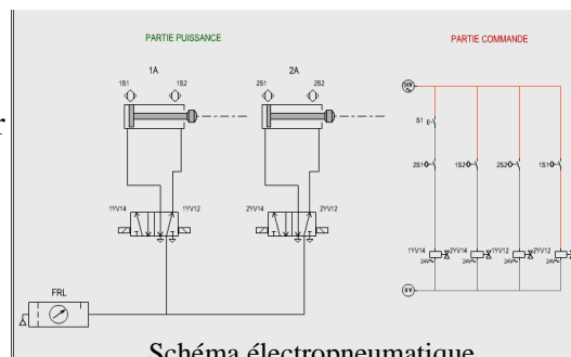
Schéma électropneumatique Réalisé par un élève
